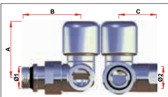
* = con testina termostatica Apr.1827 Арт. 0101-0111-0102-0112
