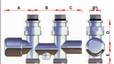
* = con testina termostatica Apr.1827 Арт. 0268
