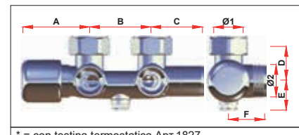
* = con testina termostatica Apr.1827 Арт. 0261
