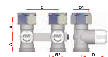
Арт. 1423-1424 Код Ø1 Ø2 A B C D 1423 G3/4 G3/4 24 33 50 40 1424 G3/4 24×19 26 33 50 40
