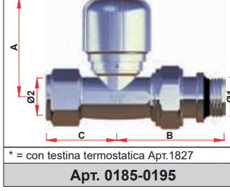
* = con testina termostatica Apr.1827 Арт. 0185-0195
