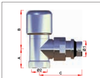
* = con testina termostatica Apr.1827 Арт. 0148-0149
