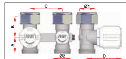
* = con testina termostatica Apt.1824 Арт. 1483-1484
