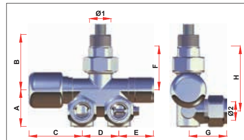
* = con testina termostatica Apr.1827 Арт. 0286-0288
