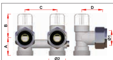
Арт. 1421-1422 Код Ø1 Ø2 A B C D 1421 G3/4 G3/4 27 37 50 33 1422 G3/4 24×19 29 37 50 33
