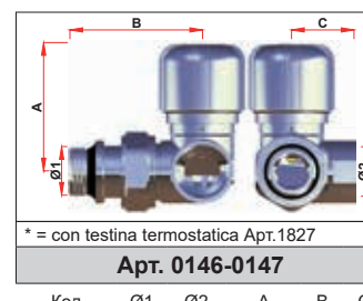
* = con testina termostatica Apr.1827 Арт. 0146-0147
