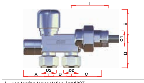
* = con testina termostatica Apr.1827 Арт. 0265
