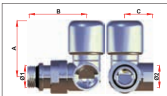
* = con testina termostatica Apr.1827 Арт. 0103-0113-0104-0114
