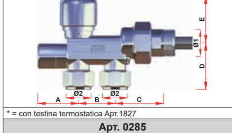
* = con testina termostatica Apr.1827 Арт. 0285
