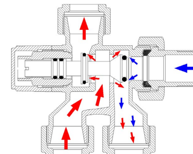
Εικ.2: Τομή διακόπτη σε θέση μονοσωληνίου (ένα μέρος της ροής διοχετεύεται στο σώμα και το υπόλοιπο στο by-pass)
